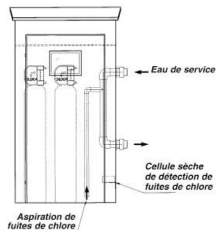
Chloromètre de sécurité CIFEC Chloro+ et dispositif d'absorption de fuites de chlore
